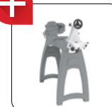
JWL-1440VS • Устройство для быстрого откидывания/установки в рабочее положение задней бабки (арт. 719001)
