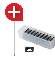
• Комплект из 10 ножей HM 15x15x2.5 мм для вала helical (арт. 1791212) • Комплект из 10 ножей HM 15x15x2.5 мм R115 KCR08 для вала helical (арт. 82019711)
